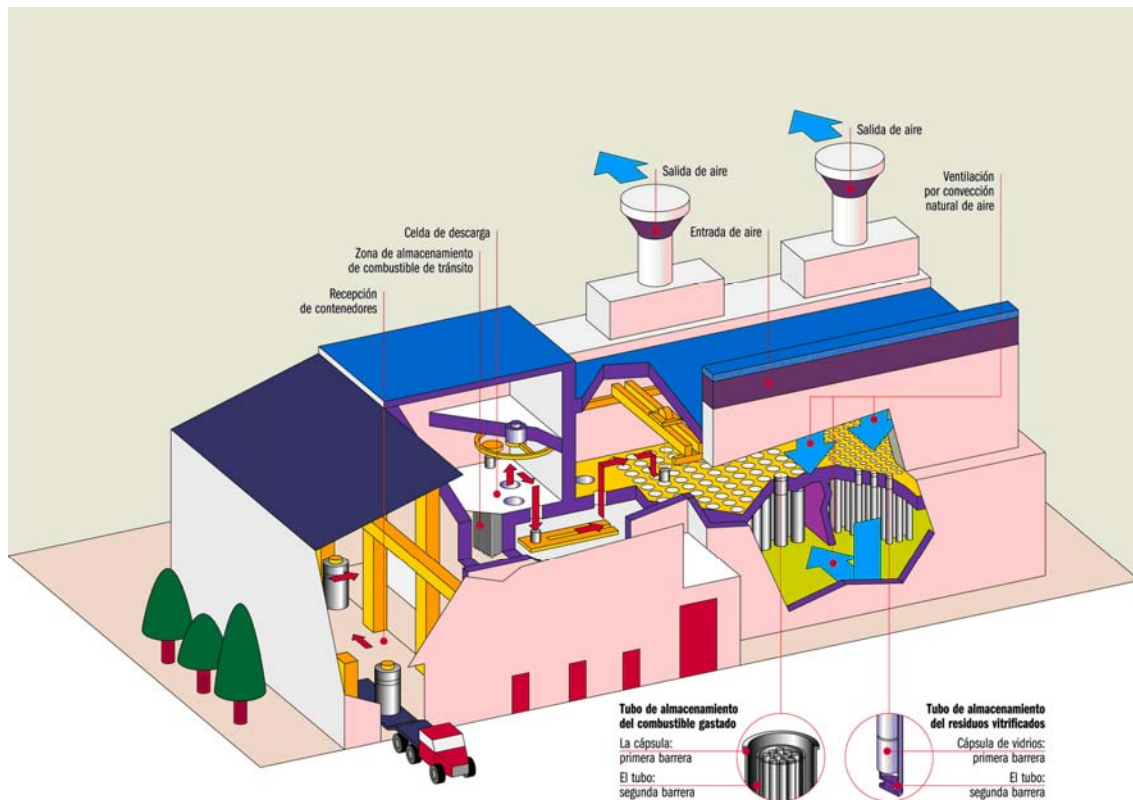
FIGURA 8. ESQUEMA ATC BÓVEDAS
