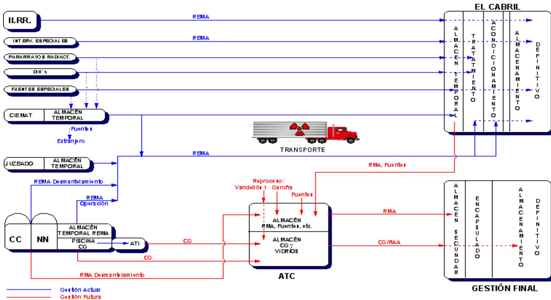
FIGURA B.2. FLUJOGRAMA GESTIÓN DE RESIDUOS RADIATIVOS EN ESPAÑA
