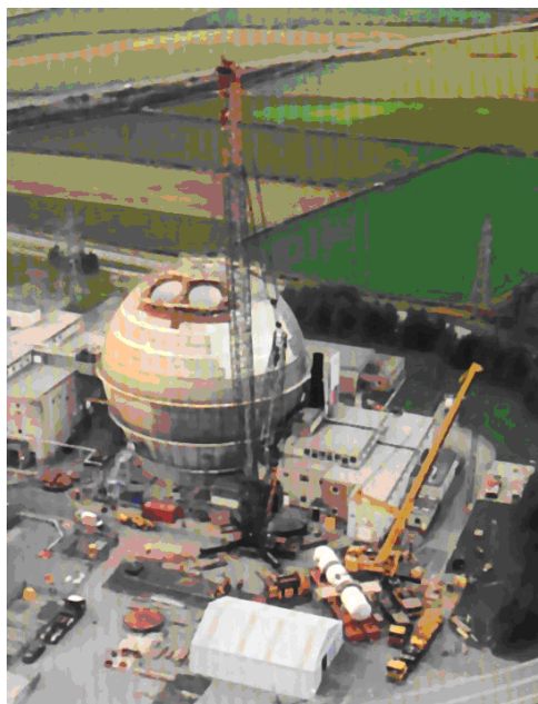
DESMANTELAMIENTO DE UNA CENTRAL TIPO AGR EN EL REINO UNIDO.
