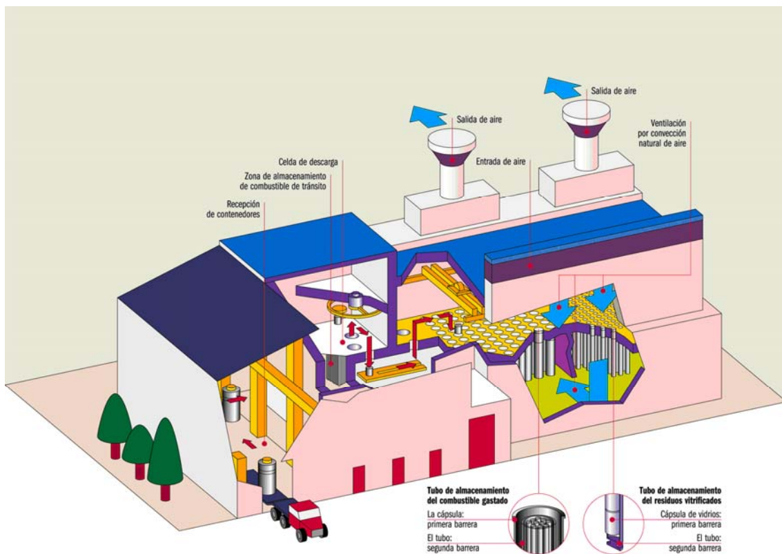
ESQUEMA ATC BÓVEDAS
