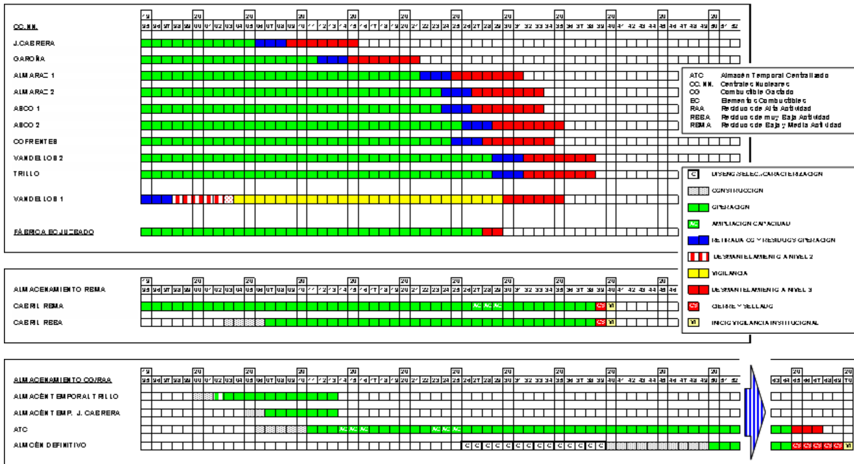
FIGURA D.2. PROGRAMA GENERAL DE LA GESTIÓN DEL COMBUSTIBLE GASTADO Y RESIDUOS RADIACTIVOS
